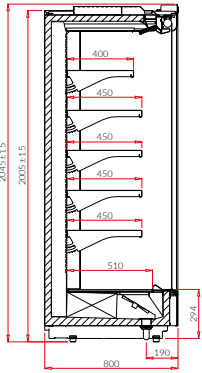
VARIO 800
