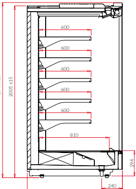
VARIO 1100
