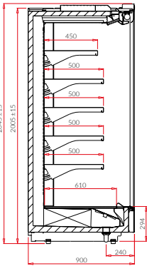
VARIO 900
