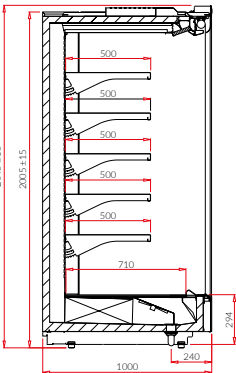
VARIO 1000
